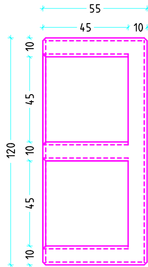
Schnitt A-A
